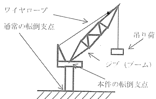
図1 本件のクレーンの構造
